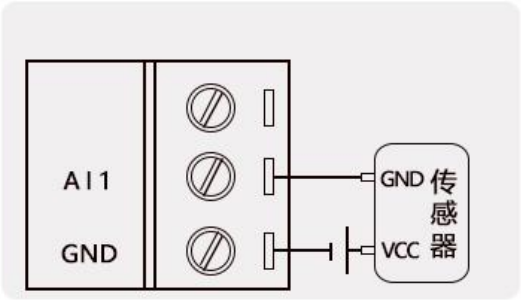
两线制传感器接线方式
