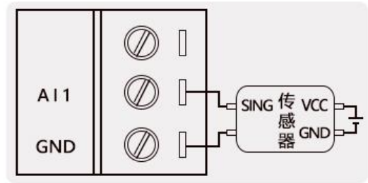
四线制传感器接线方式
