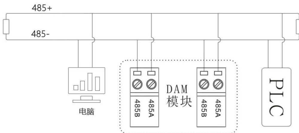
RS485组网连接示意图
