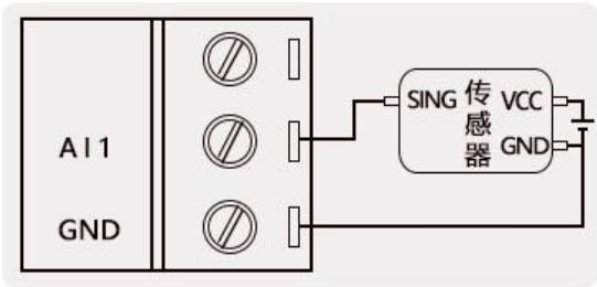
三线制传感器接线方式
