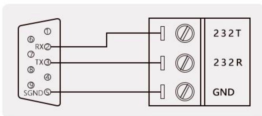
RS232接线方式
